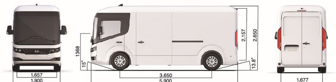
E2：外観図 単位:mm
