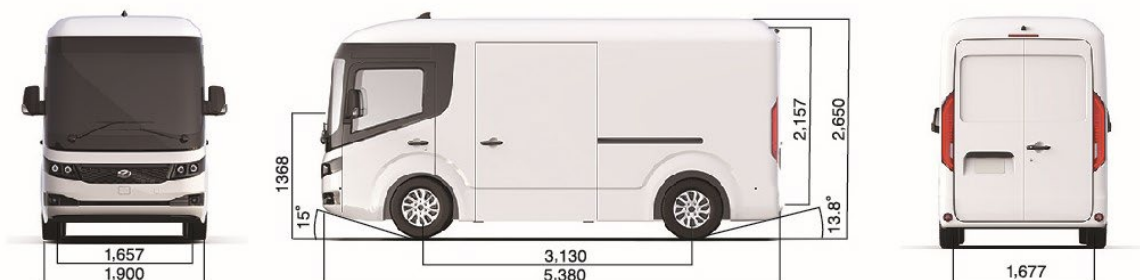
E1：外観図 単位:mm
